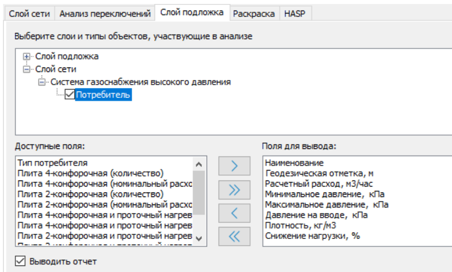
Рисунок 16.20. Настройка слоя-подложки: выбор газовой сети
