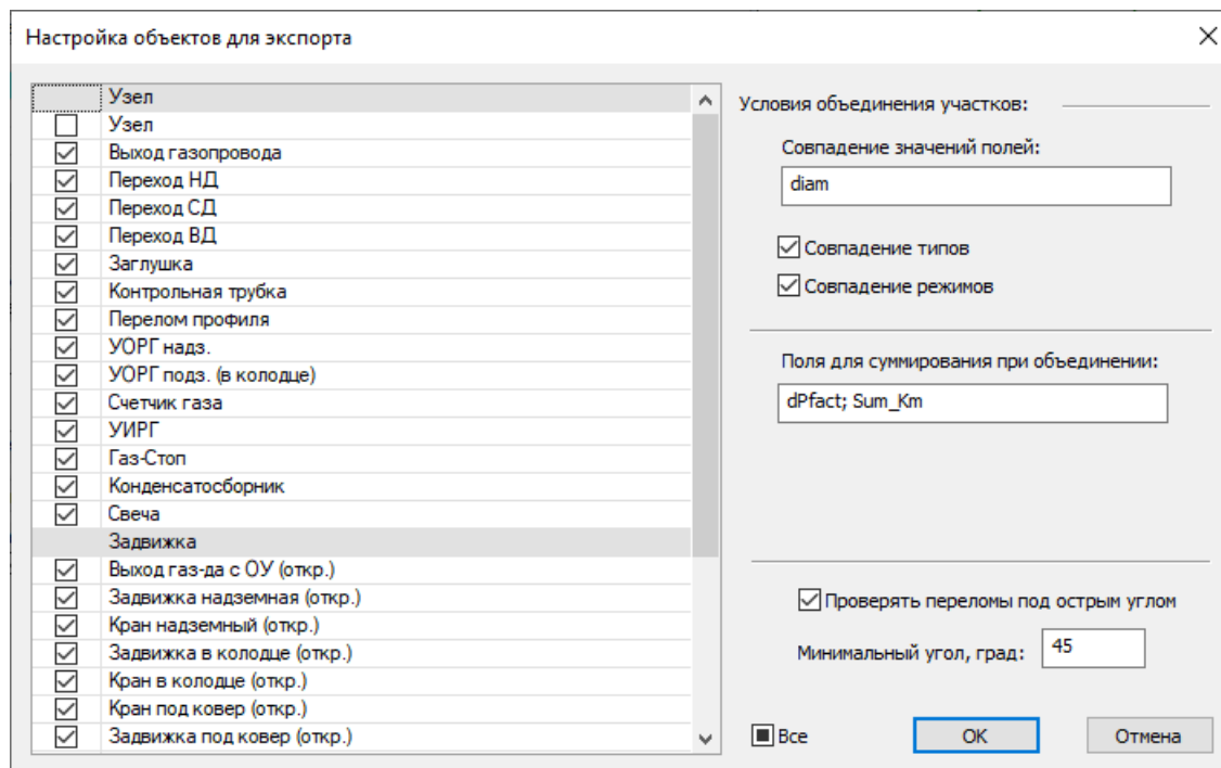
Рисунок 15.8. Настройка экспорта объектов
