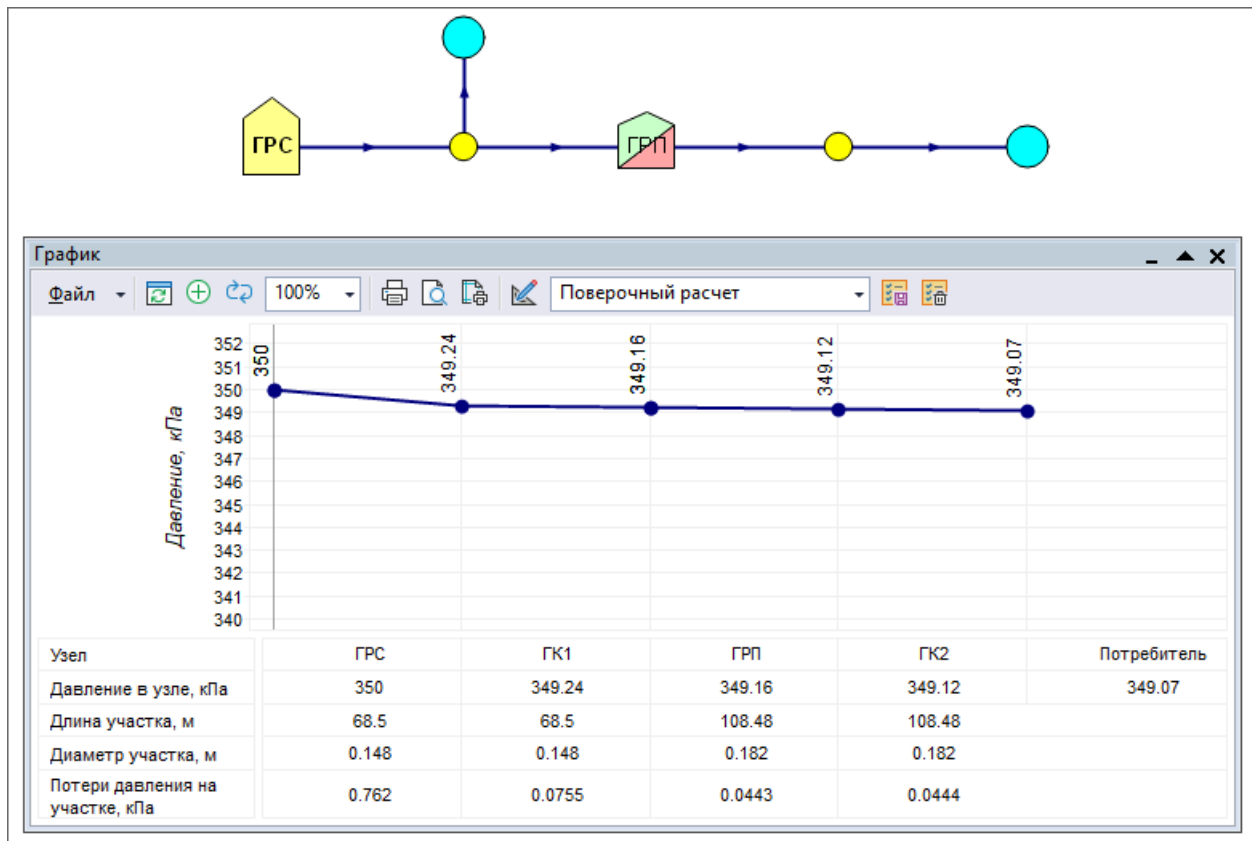
Рисунок 10.2. Пример расчета с нехваткой давления и включенной настройкой P_{out} = P_{min}
