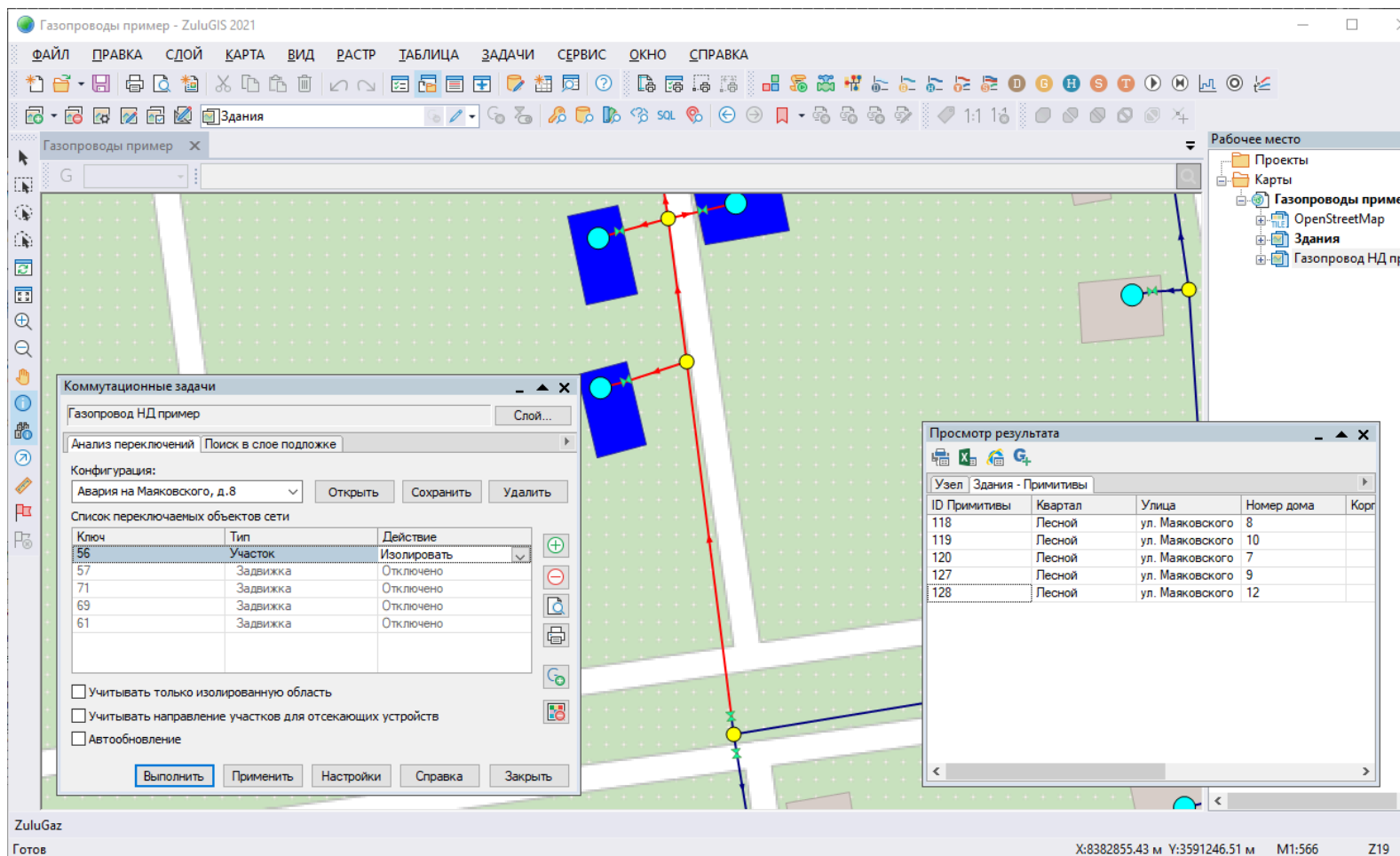
Рисунок 16.1. Пример поиска изолирующих задвижек с помощью Коммутационных задач
