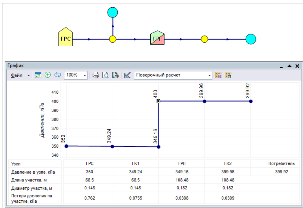
Рисунок 10.1. Пример расчета с нехваткой давления и отключенной настройкой P_{out} = P_{min}
