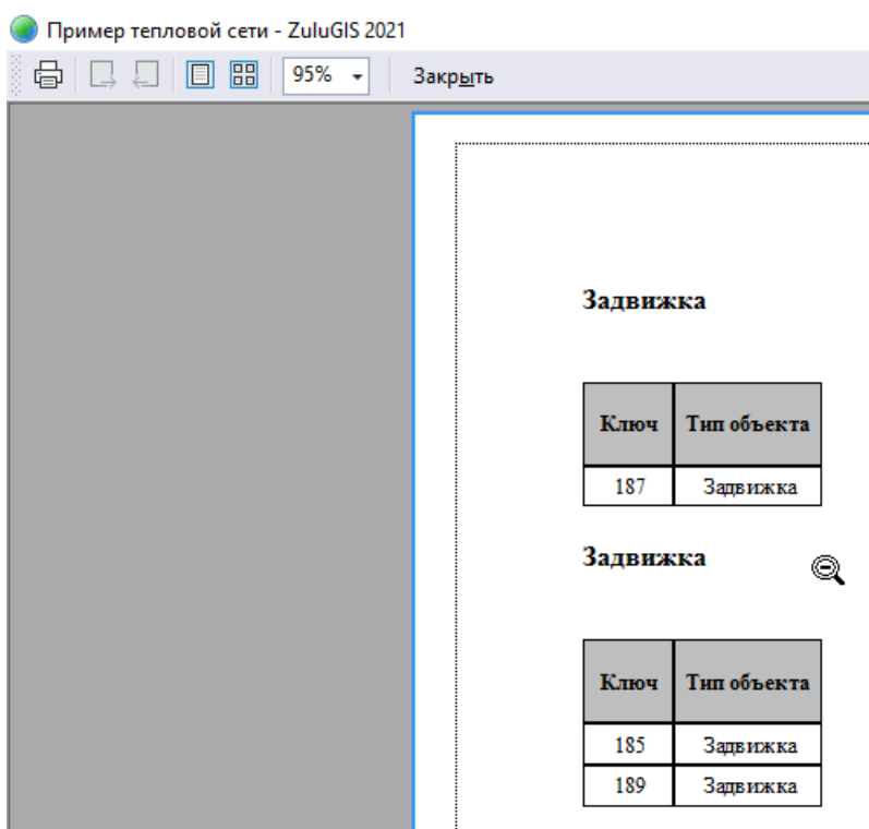
Рисунок 16.27. Отчет по списку отключаемых объектов
