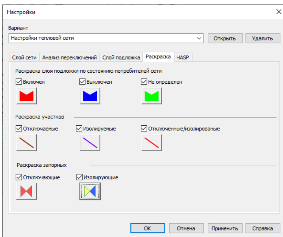
Рисунок 16.21. Настройка раскраски слоя подложки
